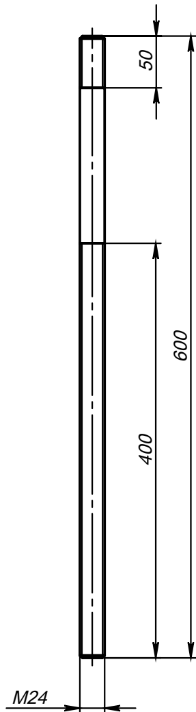
Поз.5 (Шпилька)
